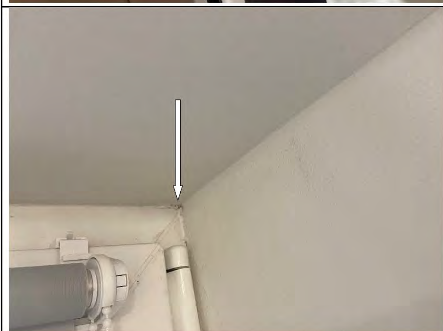
Фото №62. Неровности, выбоины, раковины на окрашенных откосах оконного блока ПВХ в спальне.
