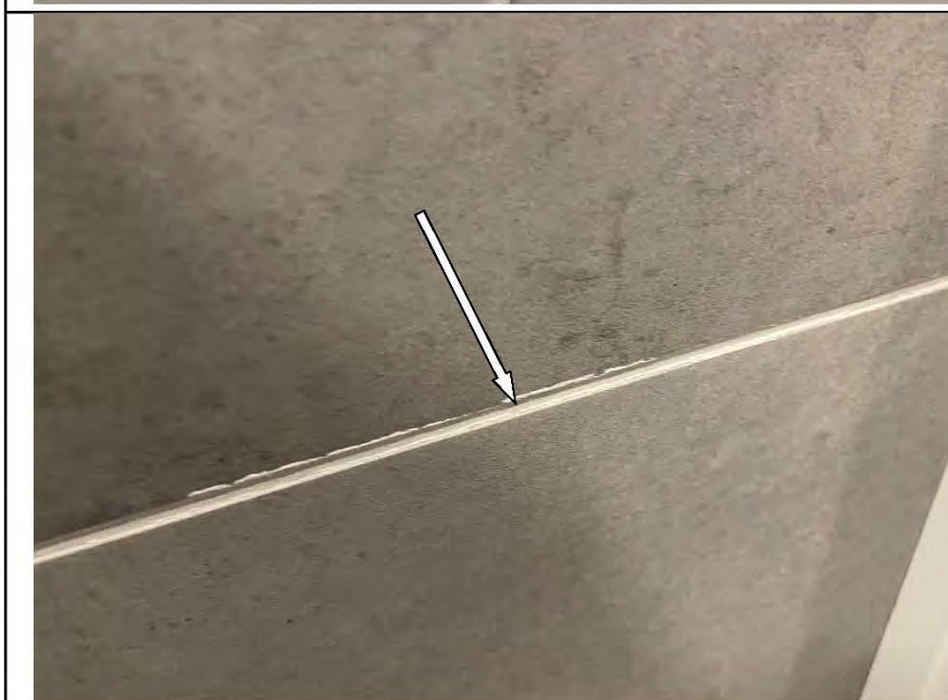
Фото №20. Неровные швы настенной керамической плитки в санузле.
