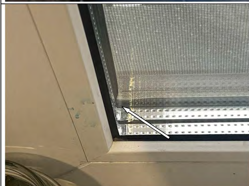
Фото №71. Дефект на уплотнительной ленте оконного блока ПВХ в спальне.
