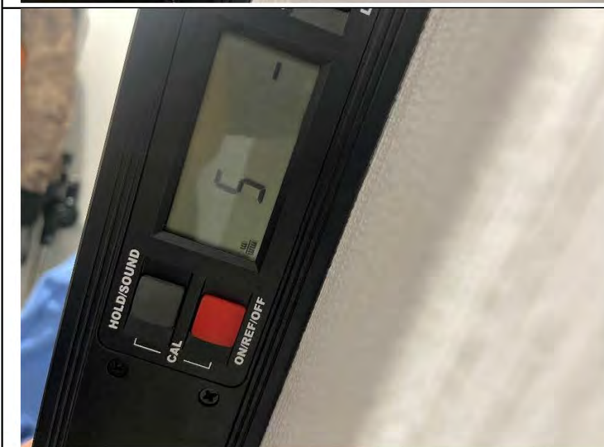
Фото №12. Отклонение поверхности стен от вертикали в кладовой.
